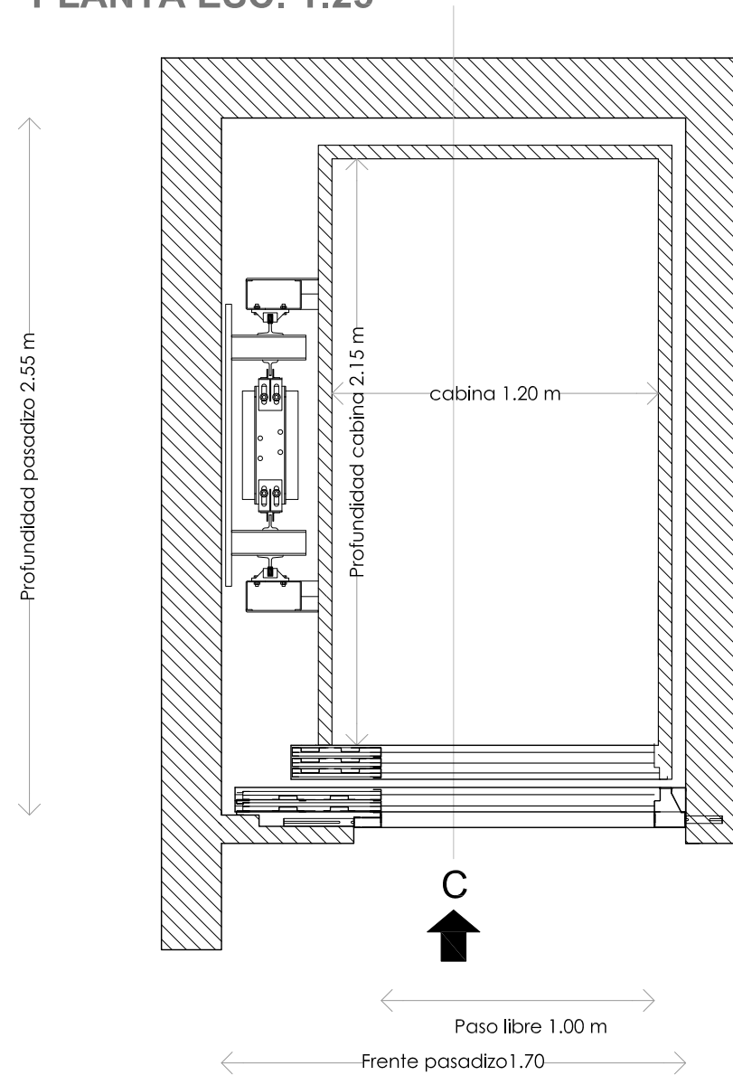
PLANTA ESC: 1:25
