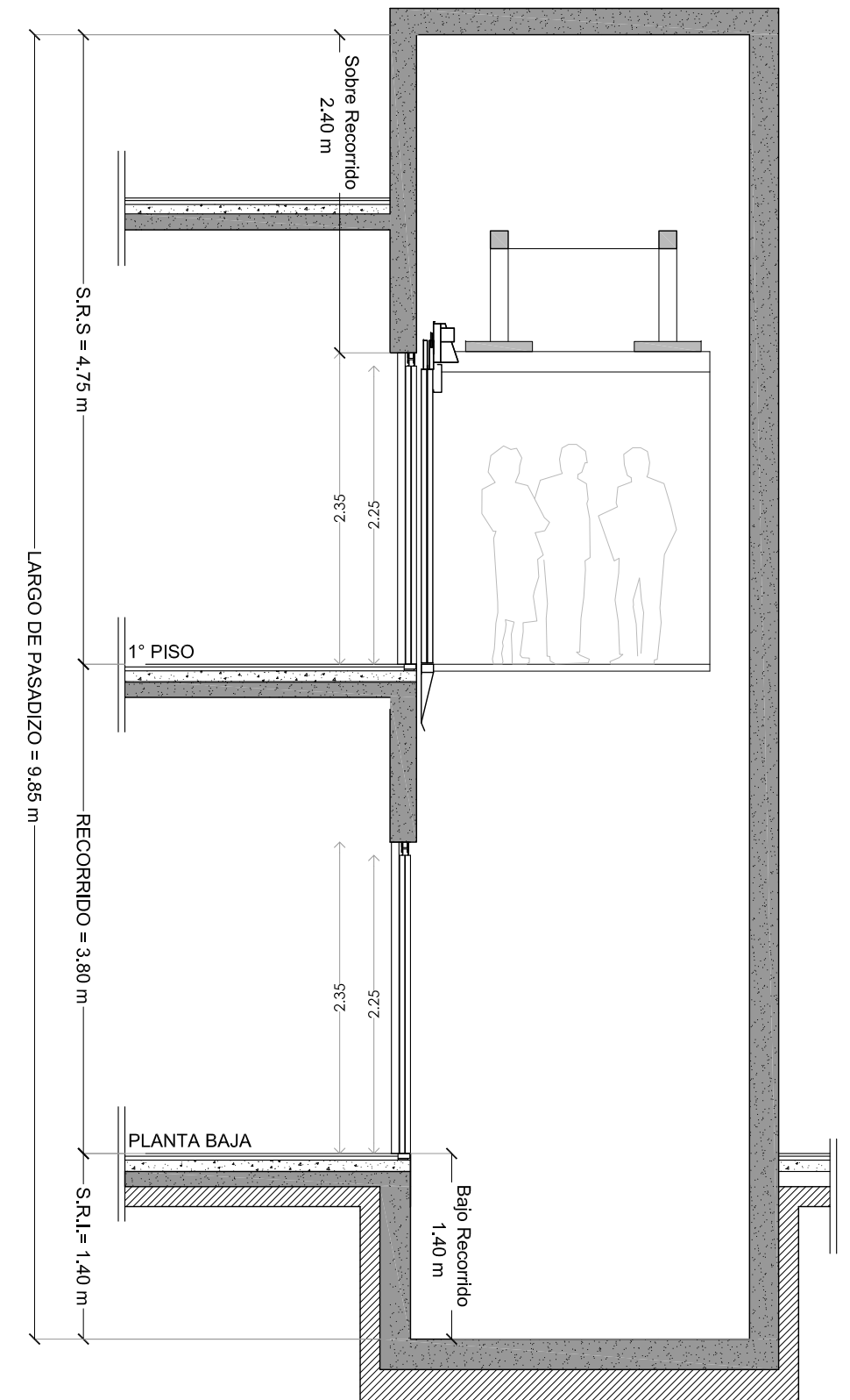
CORTE ESC: 1:50
