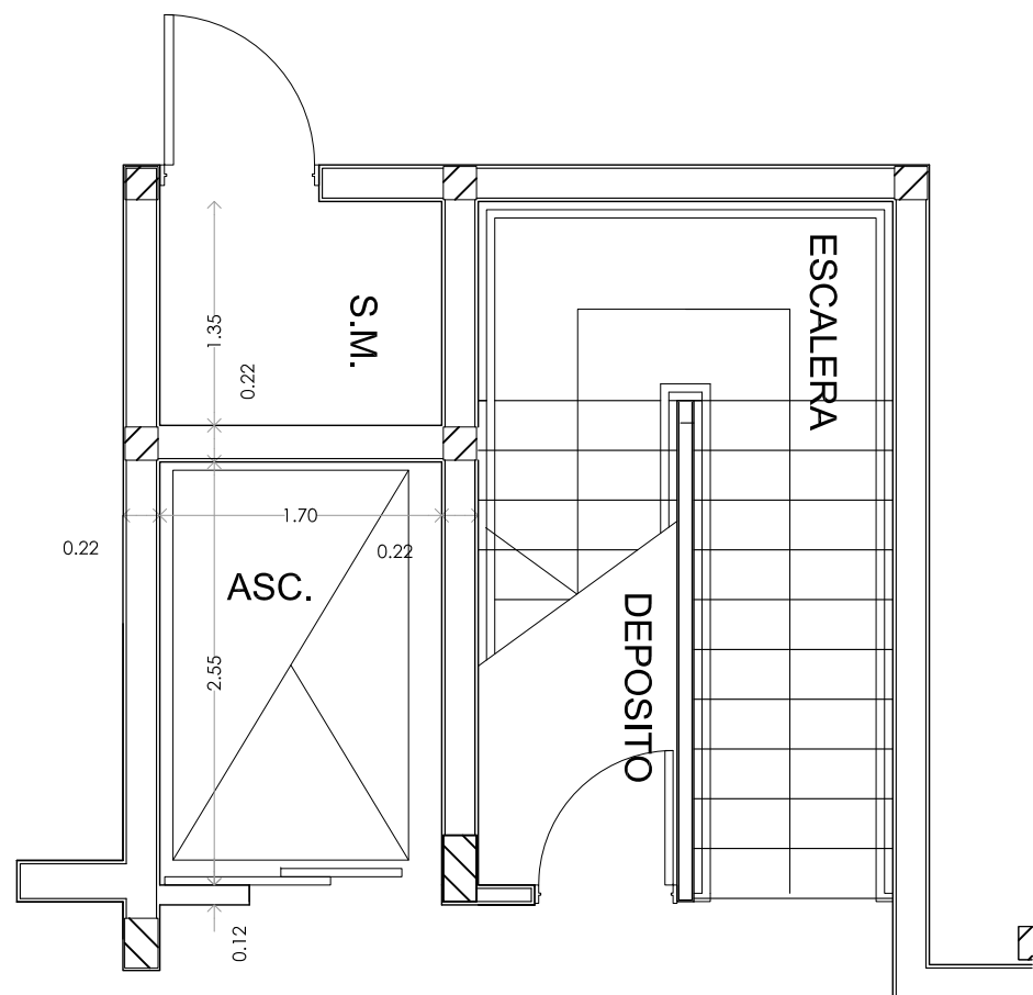
PLANTA ESC: 1:50
