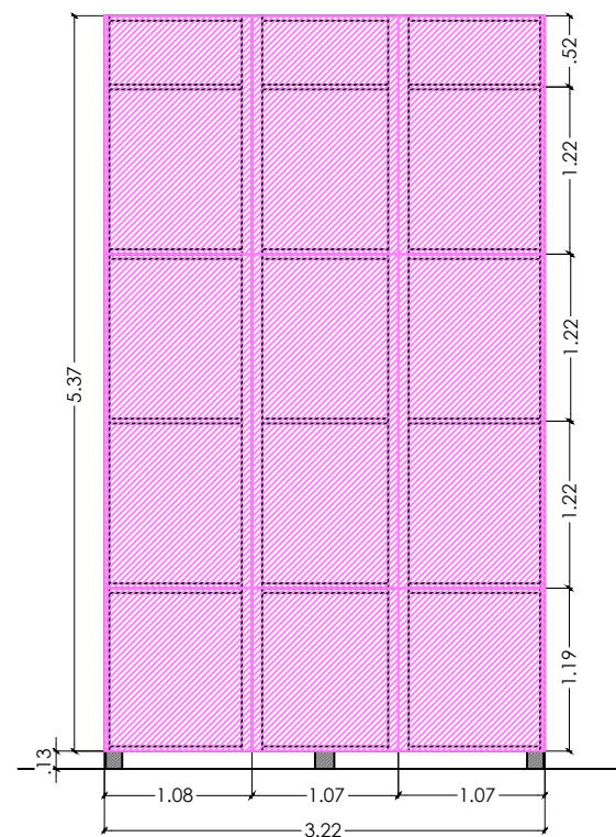
PLACAS OSB DE 9MM DE BASE SOBRE PERFILERIA GALVANIZADA
