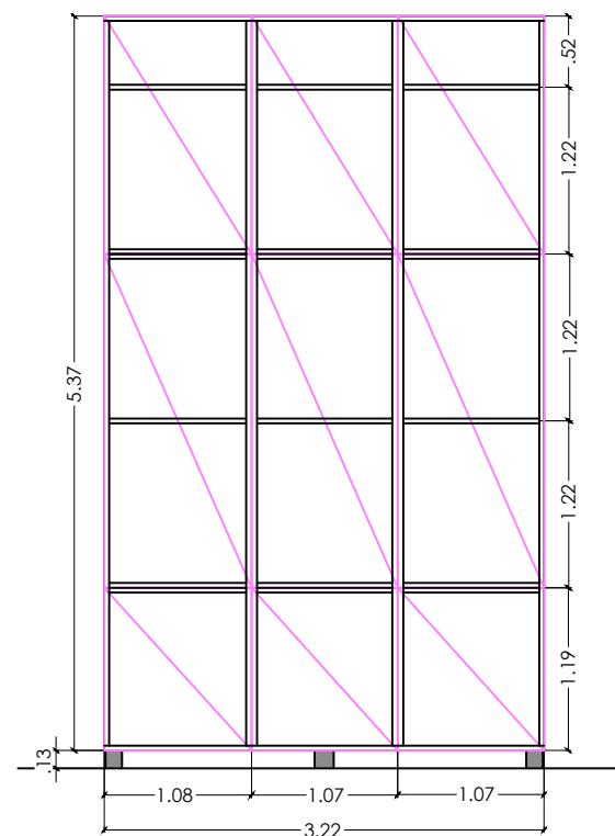
CHAPAS GALVANIZADAS SOBRE ESTRUCTURA DE PERFILERIA GALVANIZADA
