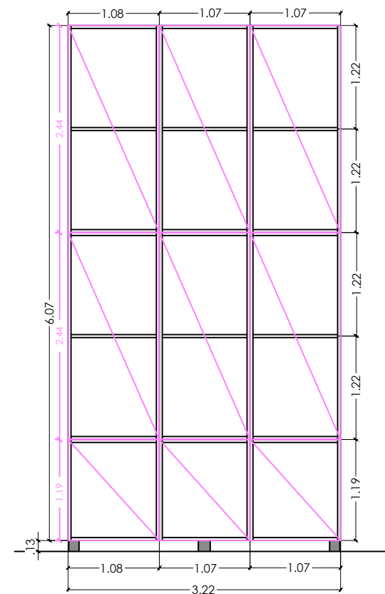
CHAPAS GALVANIZADAS SOBRE ESTRUCTURA DE PERFILERIA GALVANIZADA
