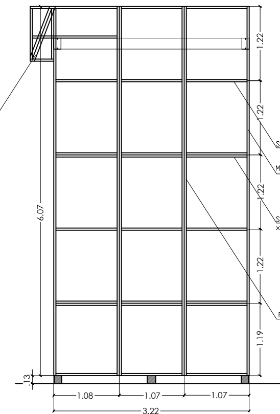
ESTRUCTURA STEEL FRAME PGC 140, PGU 140 Y PGC 90
