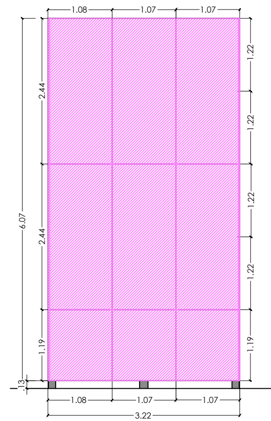
PLACAS OSB DE 9MM DE BASE SOBRE PERFILERIA GALVANIZADA
