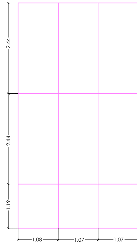
CHAPAS GALVANIZADAS UNION POR SOLAPE PLEGADO SOBRE PLACAS DE OSB
