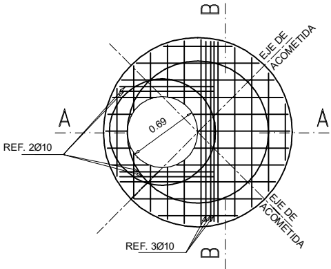
PLANTA POR E-E
