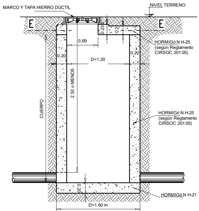
CORTE POR A-A
