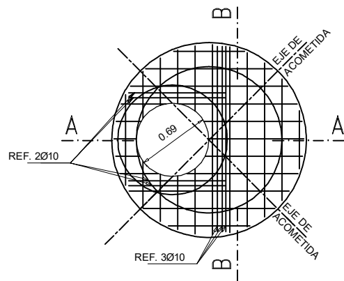
PLANTA POR E-E
