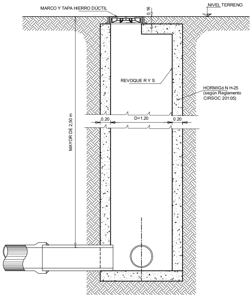
CORTE POR A-A
